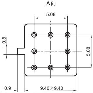
(底视图)
