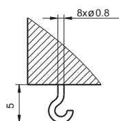
引出端形式 4 (焊钩式)
