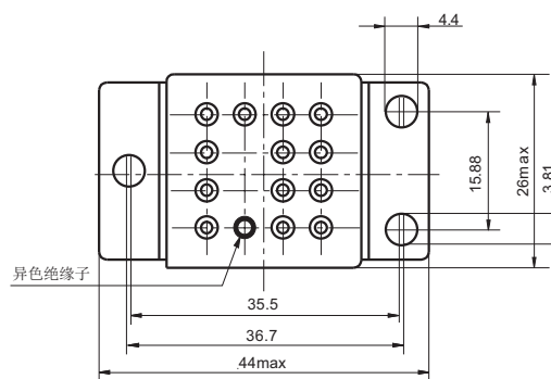
安装方式2
