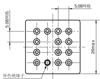
安装方式0
