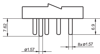
引出端形式2 (焊针式)
