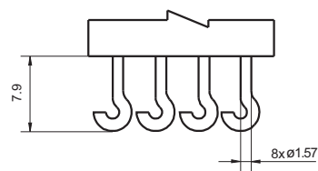
引出端形式4 (焊钩式)
