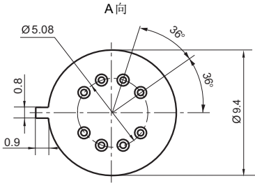
(底视图)
