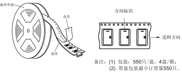
载带外形图
