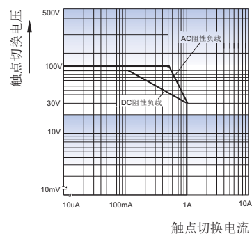
最大切换功率曲线
