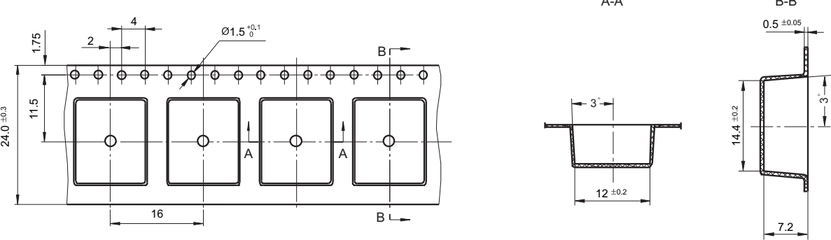
载带外形图
