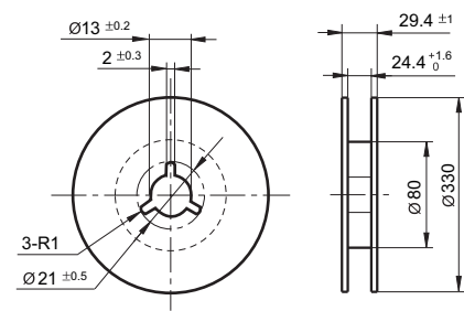
料盘外形图
