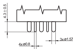
引出端形式1 (焊针式)
