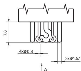
A向
