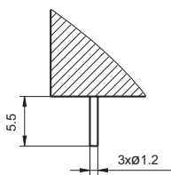
触点引出端形式 1 (焊针式)
