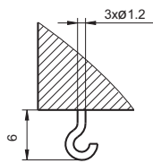
触点引出端形式 4 (焊钩式)
