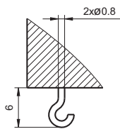
线圈引出端形式 4 (焊钩式)
