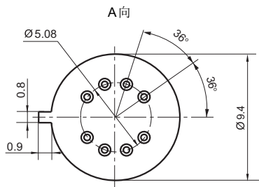
(底视图)
