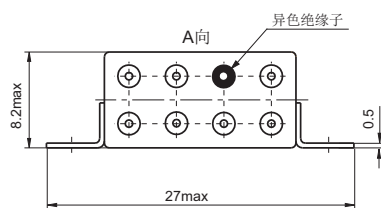
安装方式 3
