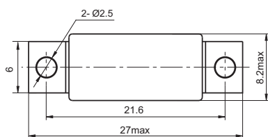
安装方式 2
