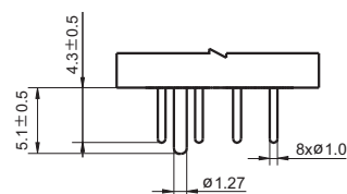
引出端形式1 (焊针式)
