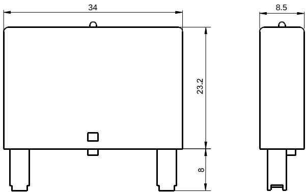
外形尺寸图
