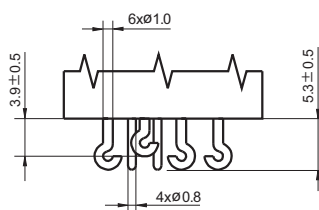
引出端形式4 (焊钩式)
