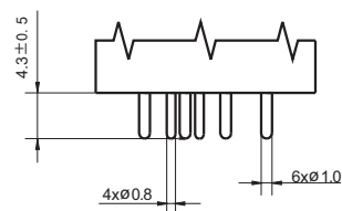
引出端形式1 (焊针式)
