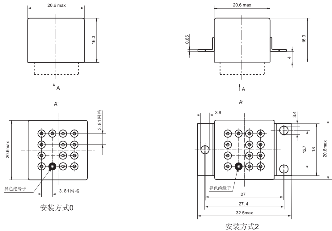
外形图
