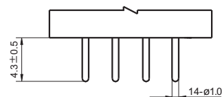
引出端形式1 (焊针式)
