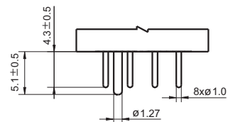
引出端形式1 (焊针式)
