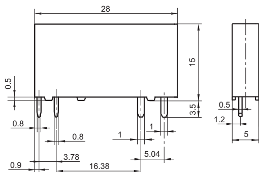
一组常开 (414)特性号
