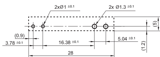
水平安装型
