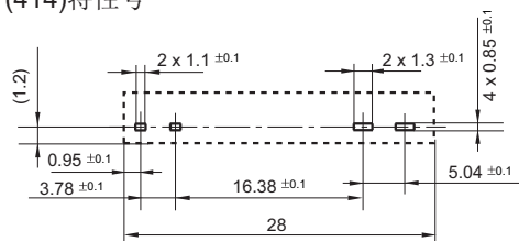
(414)特性号
