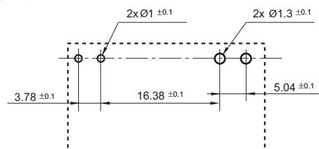
水平安装型
