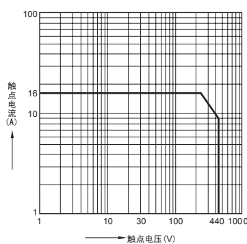
1. 通断容量的最大值 (AC电阻负载)
