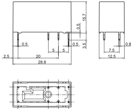
外形尺寸图
