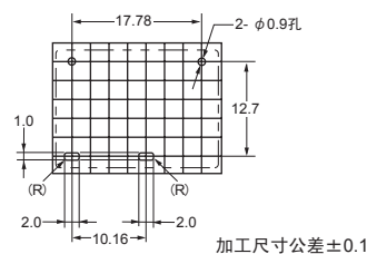
印刷板加工图 (BOTTOM VIEW)
