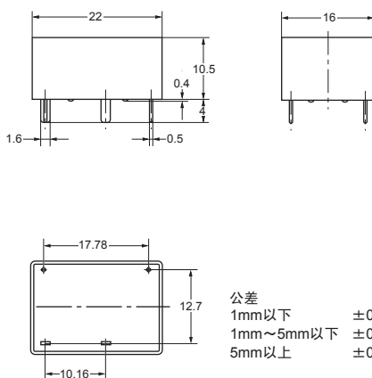
外形尺寸图
