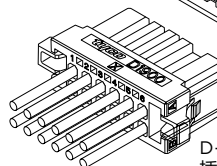
D-1900D 线路板安装水平式 (P.25 参照)
