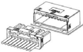
线路板安装水平式 (P.14)
