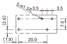
RJ1V 基准型 (SPDT)
