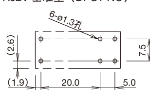
RJ1V 大容量型 (SPST-NO) RJ2V 基准型 (DPST-NO)
